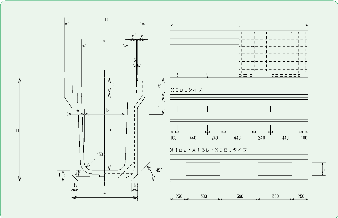
寸法・重量表
